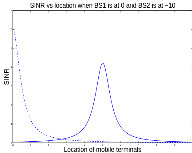
Figure 10: SINR comme fonction de l'ubication de terminal mobiles quand BS_1 est dans la position 0 (ligne plaine) et BS_2 dans -10 (ligne en pointillés).
